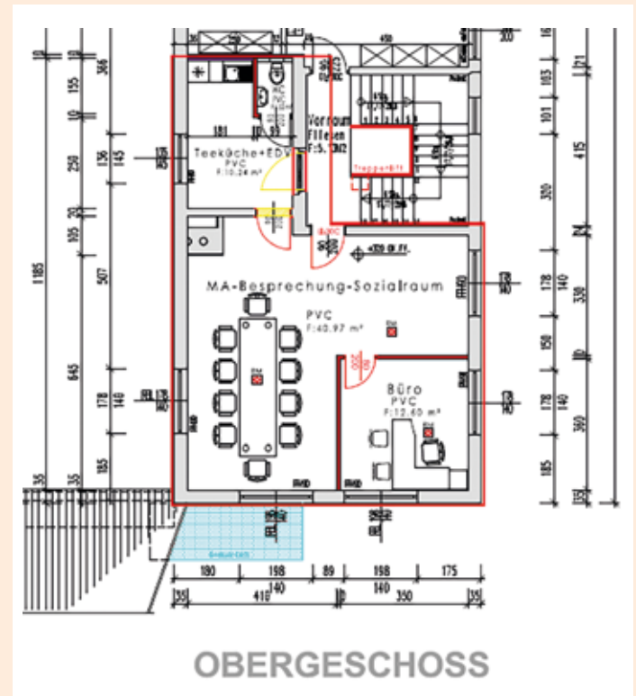
Planansicht der Mietfläche im „Ärztehaus“ (Foto: Marktgemeinde Groß Sankt Florian)
